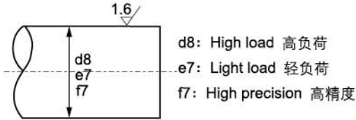
Mating Shaft 相配轴
