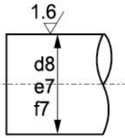
Mating Shaft 相配轴
